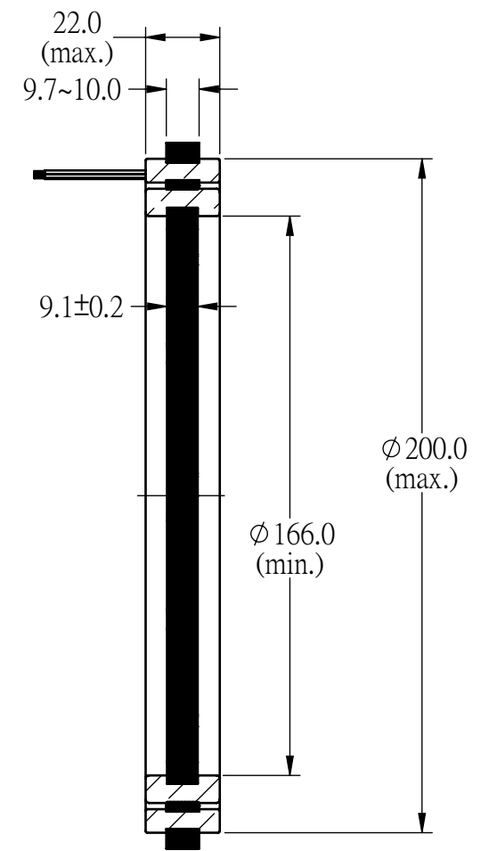
剖面圖 B-B
